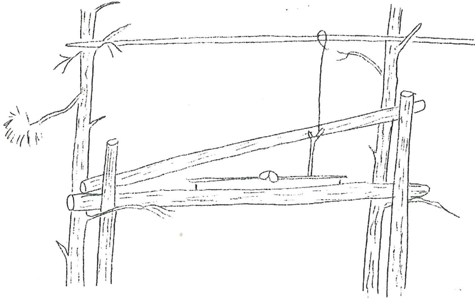
Fig. 7 a. Mårdfälla.
